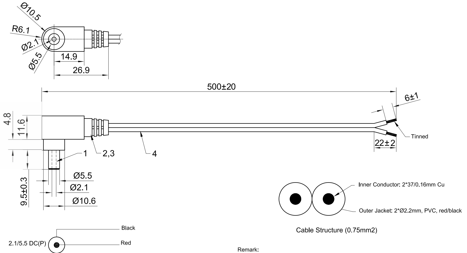
Wiring
