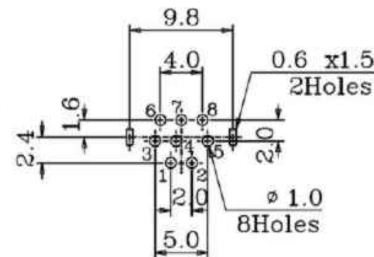
P.C.B. HOLE LAYOUT
