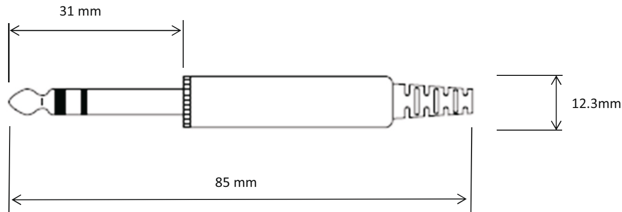
3 pin stereo plug 6,3
