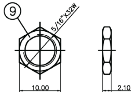
NUT
