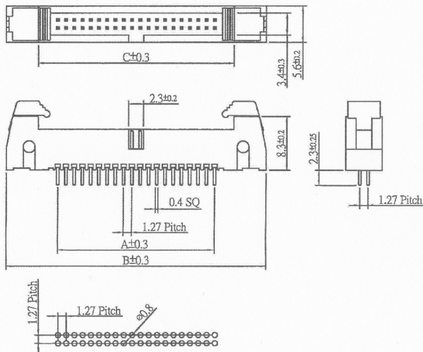
P.C.Board Layout
