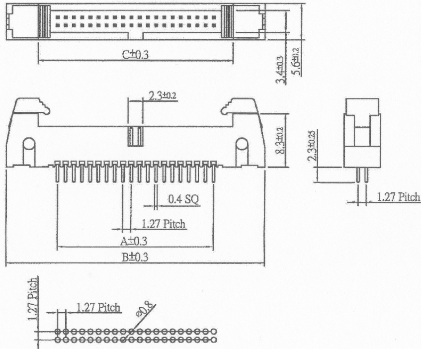
P.C.Board Layout
